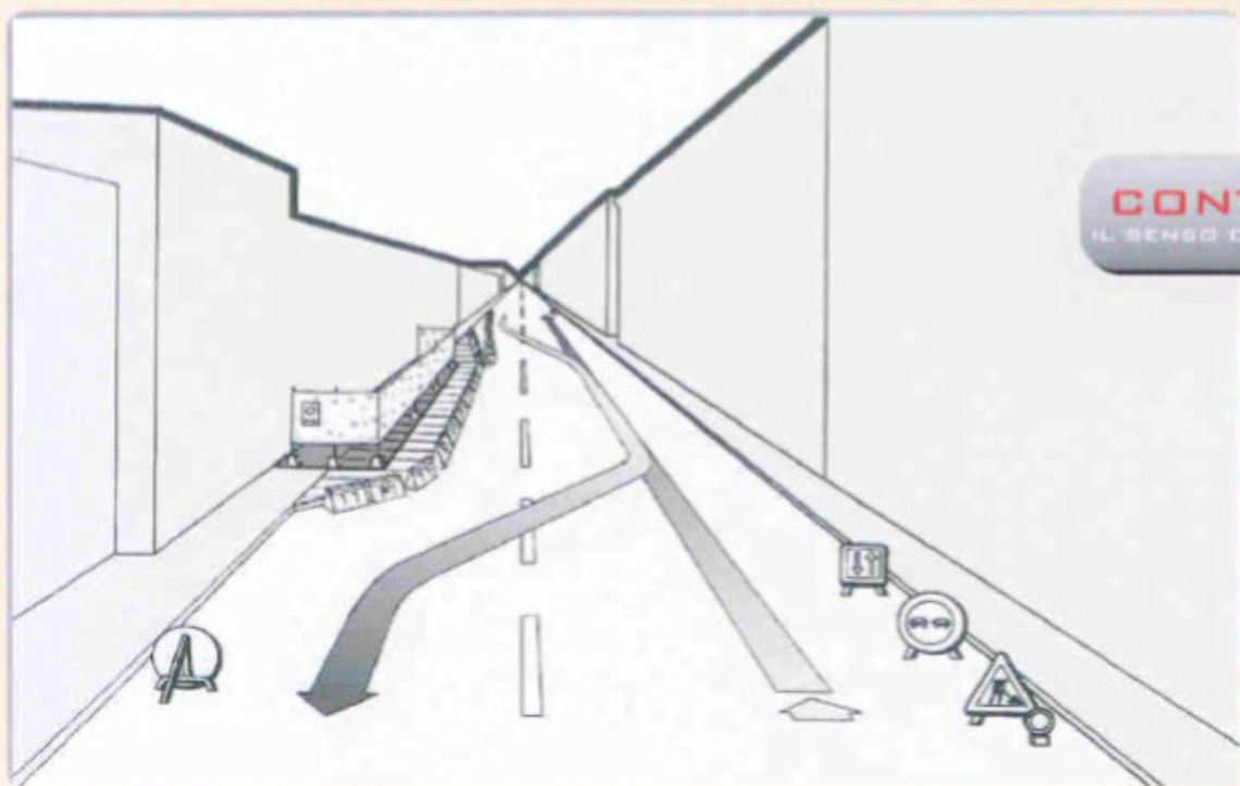
+ Figura 7a Carreggiata libera minore di 5,60 m e larghezza corsia libera dai lavori maggiore di 2,75 m con passaggi
