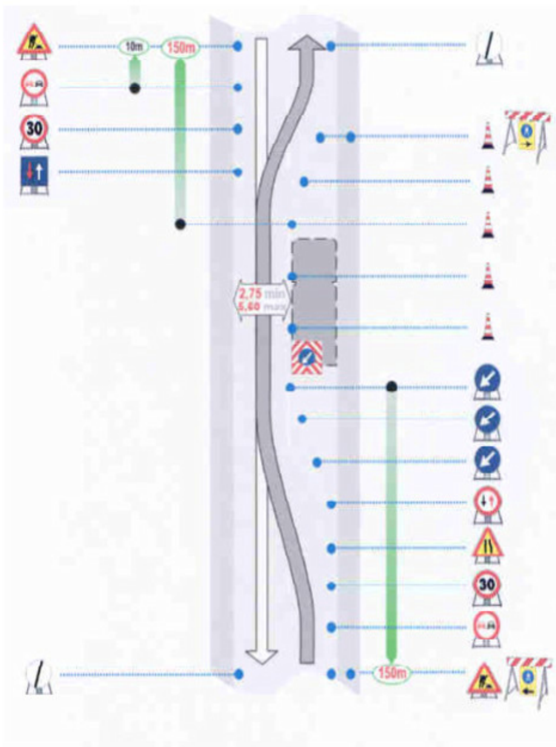
Figura 5b – Carreggiata libera minore di 5,60 m e larghezza corsia libera dai lavori maggiore di 2,75 m con presenza di automezzi con cestelli elevatori. Figura operativa.
