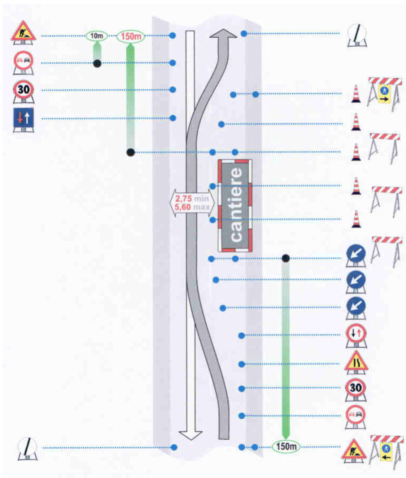
Figura 4b – Carreggiată liberă minor de 5,60 m e larghezza corsia libera dai lavori maggiore di 2,75 m. Figura operativa.
