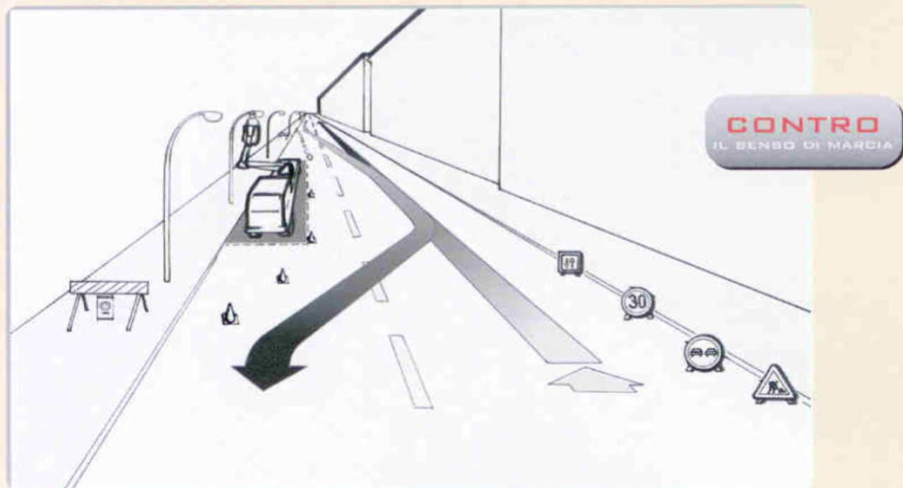
Figura 5a Carreggiata libera minore di 5,60 m e larghezza corsia libera dai lavori maggiore di 2,75 m con presenza di automezzi con cestelli elevatori. Figura descrittiva.
