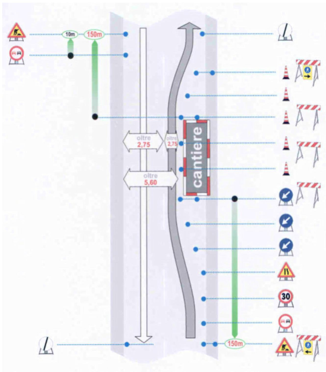
Figura 2b Carreggiata libera maggiore di 5,60 m e larghezza corsia libera dai lavori maggiore di 2,75 m. Figura operativa.
