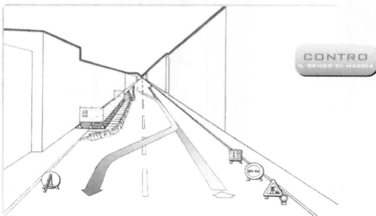
+ Figura 7a Carreggiata libera minore di 5,60 m e larghezza corsia libera dai lavori maggiore di 2,75 m con passaggi protetti per pedoni. Figura descrittiva.
