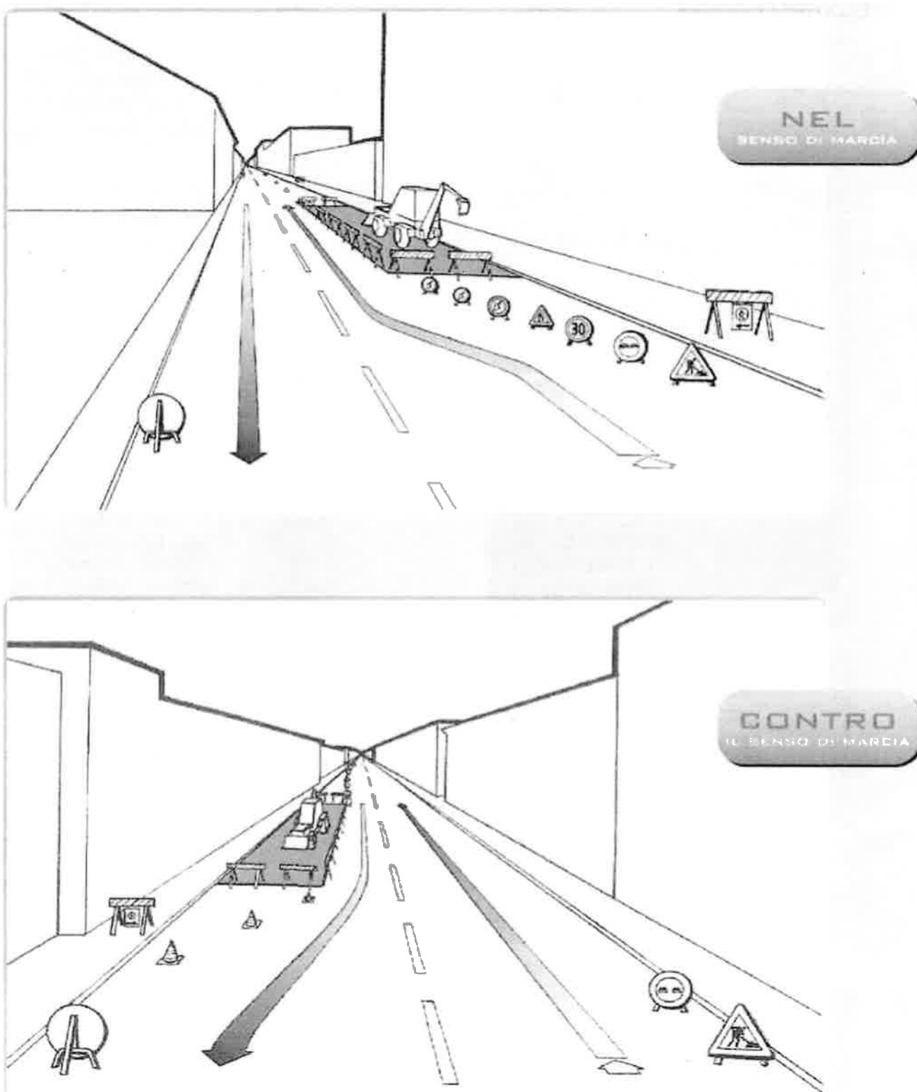
Figura 2a Carreggiata libera maggiore di 5,60 m e larghezza corsia libera dai lavori maggiore di 2,75 m. Figura descrittiva.
