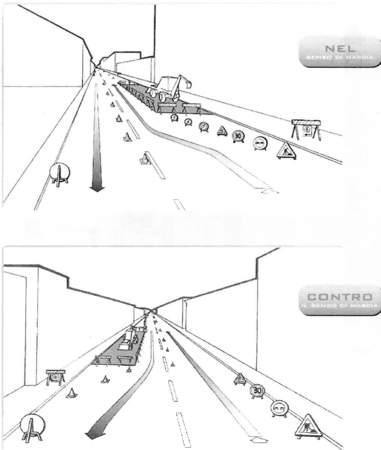
Figura 3a Carreggiata libera maggiore di 5,60 m e larghezza corsia libera dai lavori minore di 2,75 m. Figura descrittiva.
